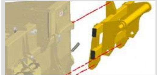
Zwischenadapter für andere Träger auf 3 Punkt-Anbau der BAV für Frontlader, Teleskoplader...
