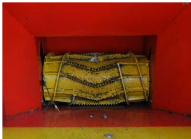
Ladetricher mit überdimensionierte Einzugswalze
